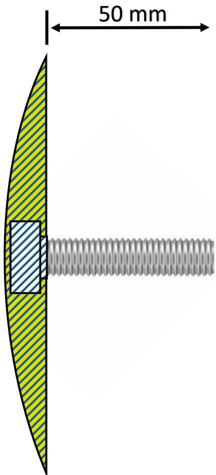
Corte Parcial
